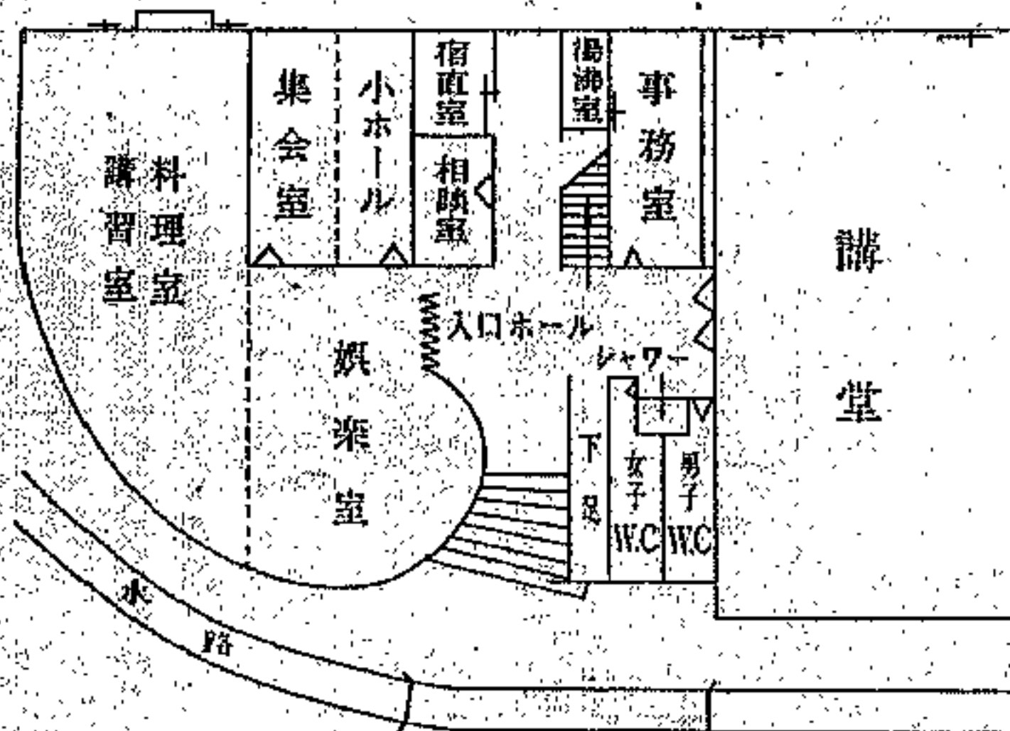
ホーム見取図(一階)
